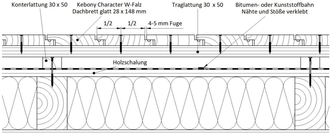
Regensicheres Unterdach mit Belüftung
